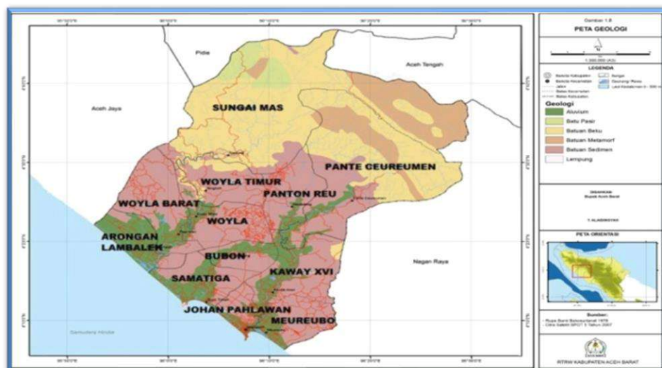
Gambar 2.3. Peta Geologi Kabupaten Aceh Barat
